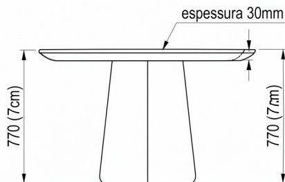
elevação frontal
